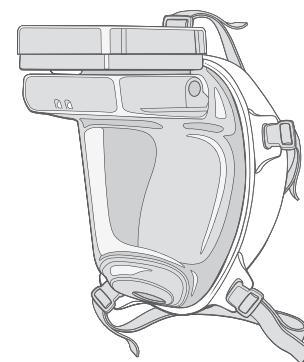
MOTORISCH BETRIEBENES LUFTREINIGENDES ATEMSCHUTZGERÄT (PAPR)
